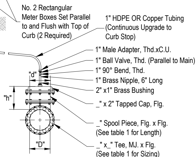
D, Nominal Diameter of Main, In. Minimum d, In. Minimum h, In. Comments 6 6.0 6.0 6" MJ x 6" MJ x 6" FLG DI TEE 8 8.0 8.0 8" MJ x 8" MJ x 8" FLG DI TEE 12 12.0 12.0 12" MJ x 12" MJ x 12" FLG DI TEE 16 12.0 9.6 16" MJ x 16" MJ x 12" FLG DI TEE 24 18.0 14.4 24" MJ x 24" MJ x 18" FLG DI TEE 30 18.0 18.0 30" MJ x 30" MJ x 18" FLG DI TEE 36 24.0 21.6 36" MJ x 36" MJ x 24" FLG DI TEE 42 24.0 25.2 42" MJ x 42" MJ x 24" FLG DI TEE 48 24.0 28.8 48" MJ x 48" MJ x 24" FLG DI TEE 54 30.0 32.4 Welded-on FLG Outlet 60 36.0 36.0 Welded-on FLG Outlet 66 24.0 23.1 Welded-on FLG Outlet 72 24.0 25.2 Welded-on FLG Outlet
